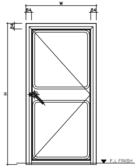
ELEVATION("B") SCALE:NONE
