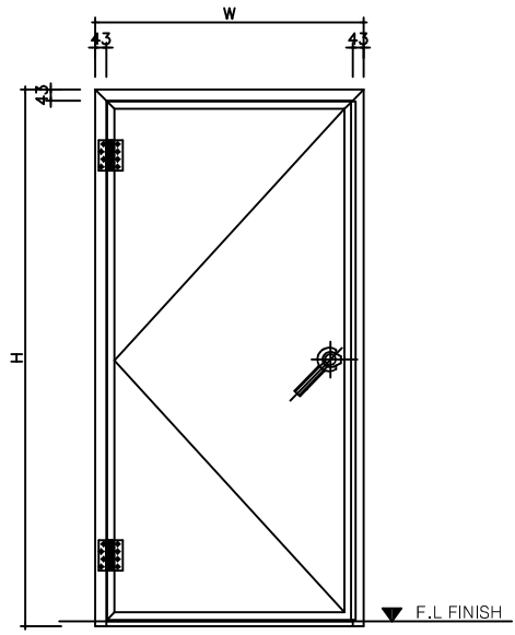
ELEVATION("A") SCALE:NONE
